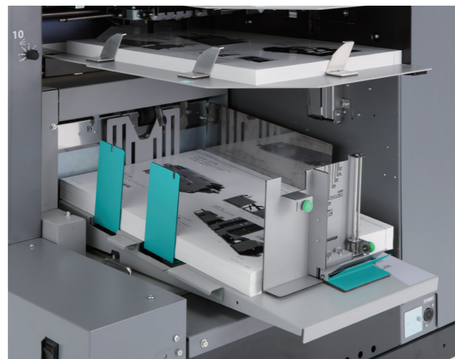
Optional stacker
